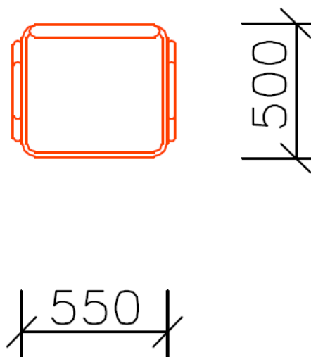
Obr. Křeslo pro studenty – horní pohled
